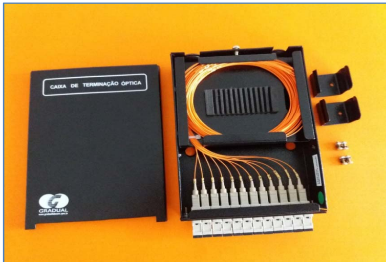
MINI DIO DIN COM 12 FIBRAS SC MM / VISTA SUPERIOR
